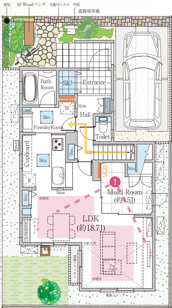
1階
