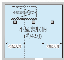
小屋裏収納
